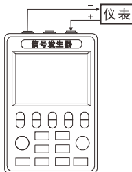
图 4 测量电压，有源电流信号
