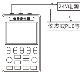
图 3 二线制变送器模拟器
