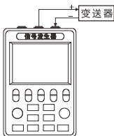
图 5 测量二线制变送器
