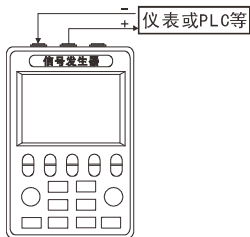
图 2 输出有源电流/电压到仪表或 PLC
