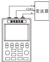
图 6 测量三线制变送器
