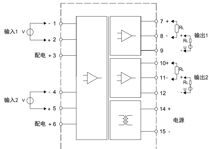
双入双出电压输入接线图
