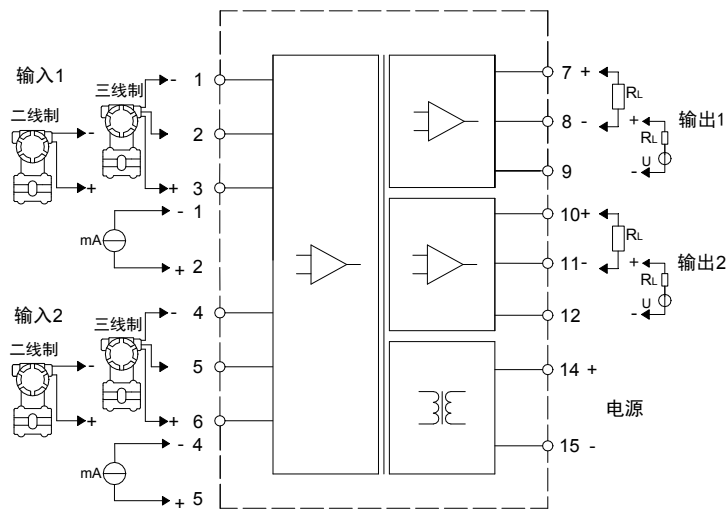
双入双出电流输入接线图
