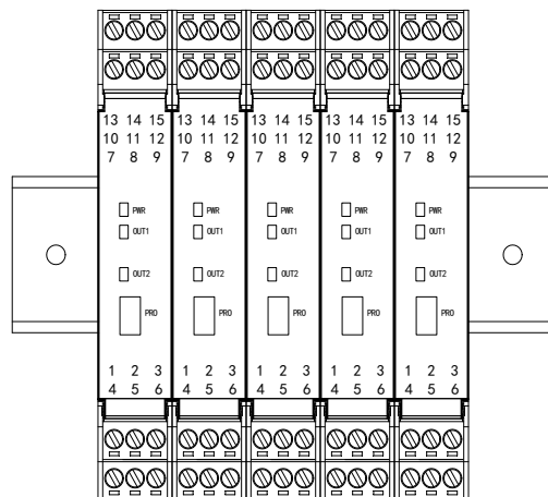
垂直安装示意图
